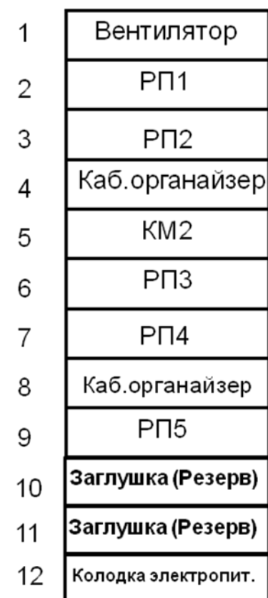
Рисунок 7. Фасад шкафа РШ2.1
